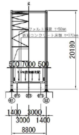
▲標準断面図
