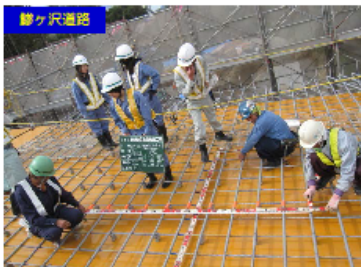
鯉ヶ沢道路 現場実習の様子
