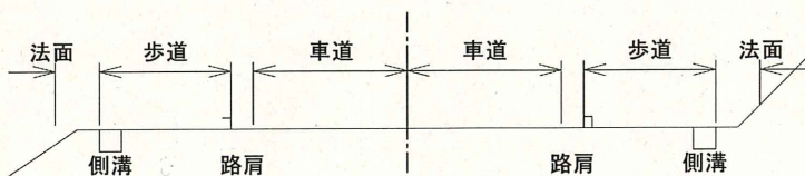
国道4号 標準断面図
