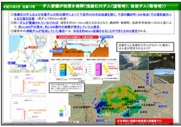
【台風18号での目屋ダム等の効果】
