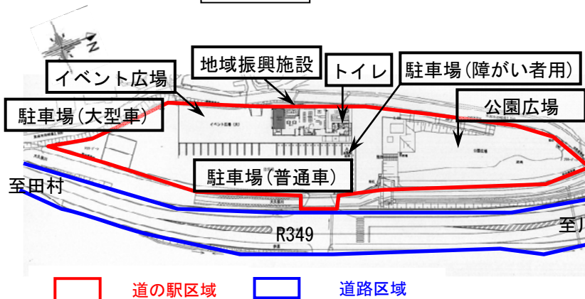
平面図
