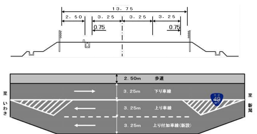
【計画断面図】
