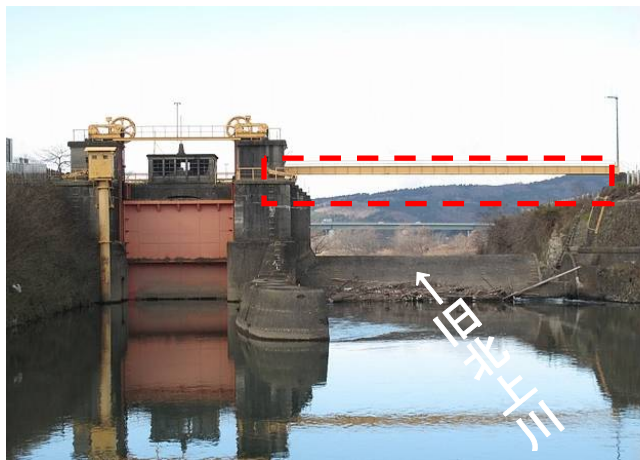
▲脇谷閘門全景(石巻市桃生町地内:北上川水系旧北上川) 【管理橋 昭和40年設置】
