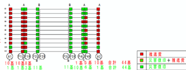
位置図 (支承)
