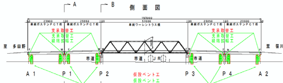
位置図 (支承)
