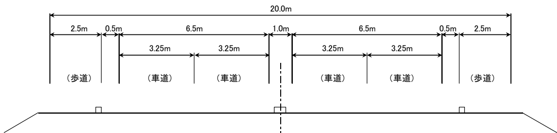
【4車完成断面】
