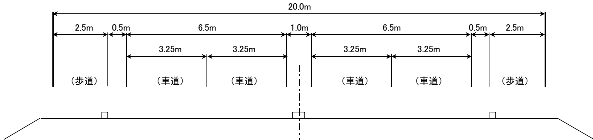
【4車完成断面】
