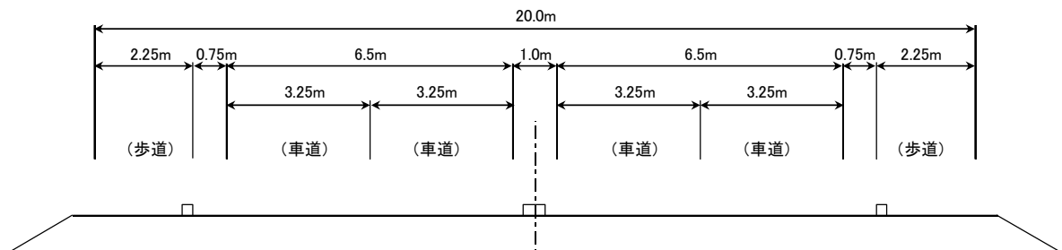
【4車完成断面】
