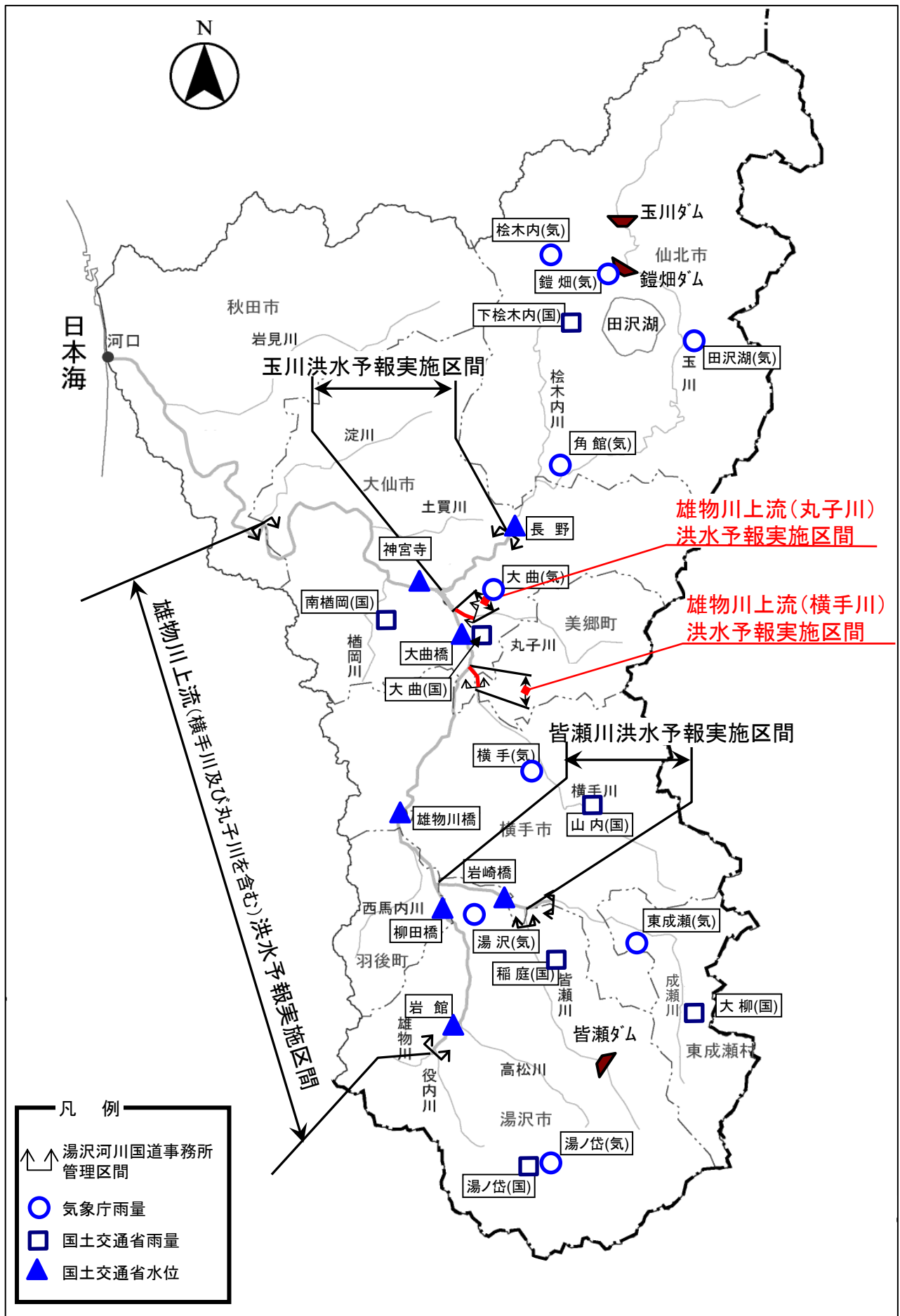
洪水予報区間及び雨量・水位観測所配置図 (雄物川上流(横手川及び丸子川含む)、皆瀬川、玉川)
