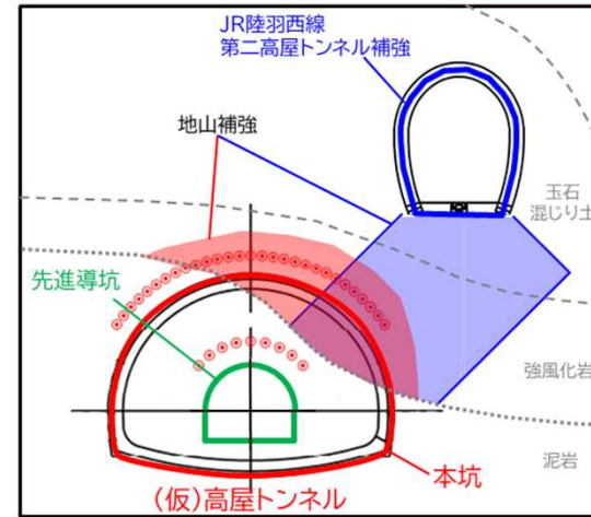
▲トンネル掘削・補強断面(A-A')
