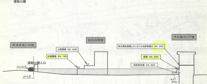
大坪川越水時総合運動公園入内一時滞留断面図
