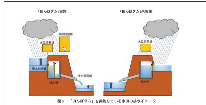
図5 「田んぼダム」を実施している水田の排水イメージ ※イメージ図は農林水産省農村振興局整備部発行資料を引用。 ※具体的な対策内容については、今後の調査・検討等により変更となる場合がある。
