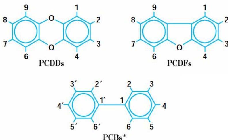
図-25 ダイオキシン類の構造図
