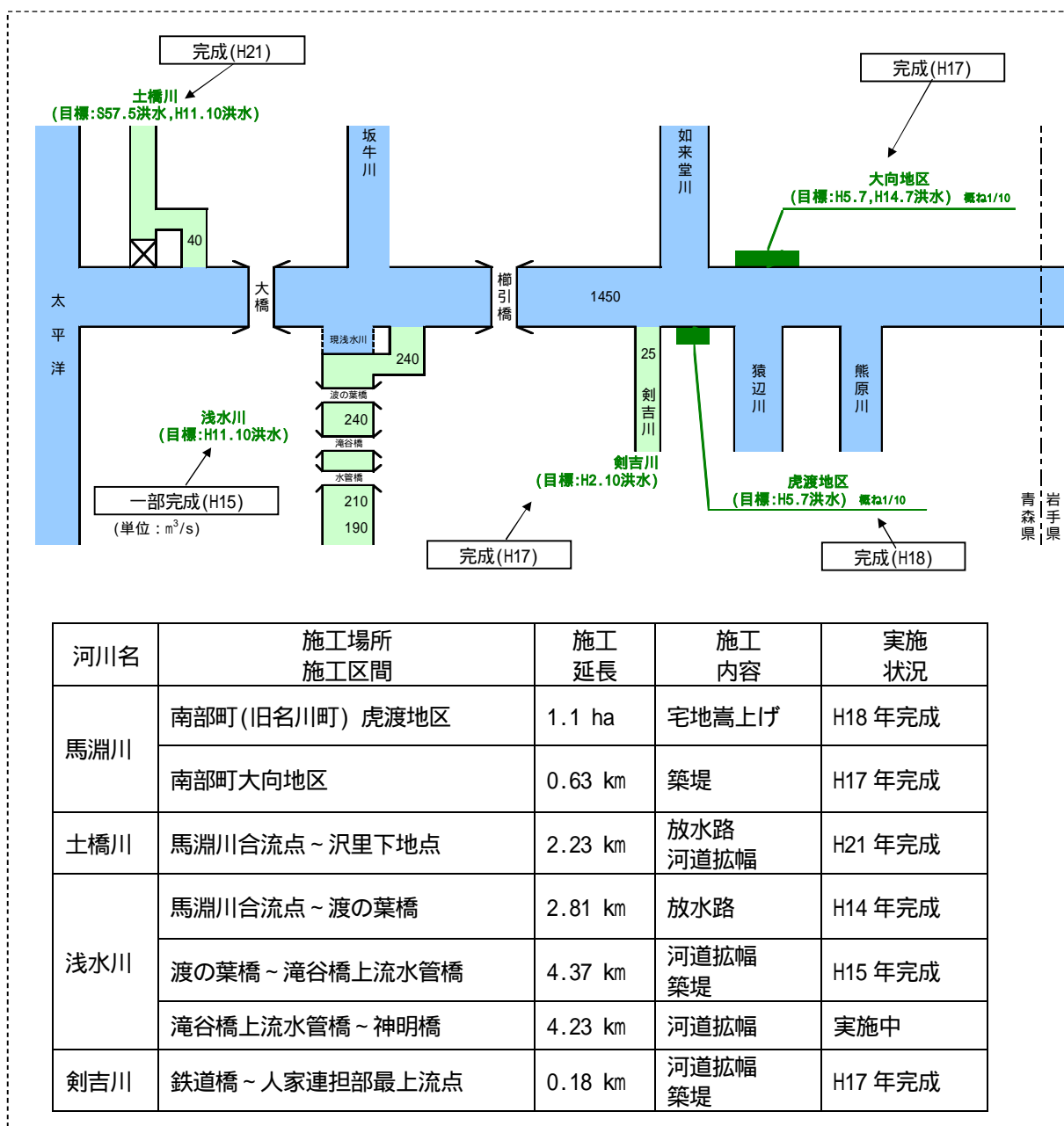
< H15.10 策定 馬淵川水系（八戸圏域）河川整備計画の目標流量と実施状況 >
