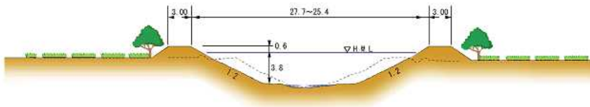
整備イメージ（横断図）
