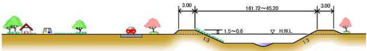
整備イメージ（馬淵川合流点～渡の葉橋の放水路）
