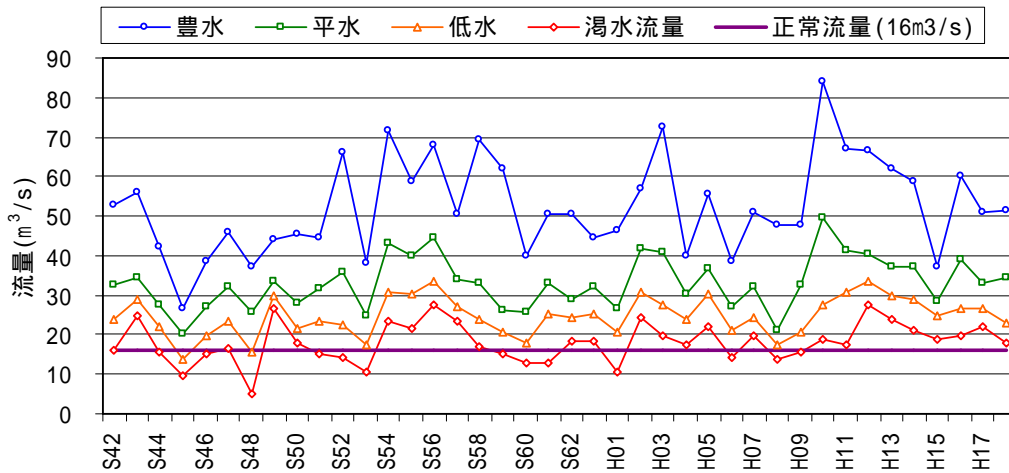
< 剣吉地点 流況の経年変化 >
