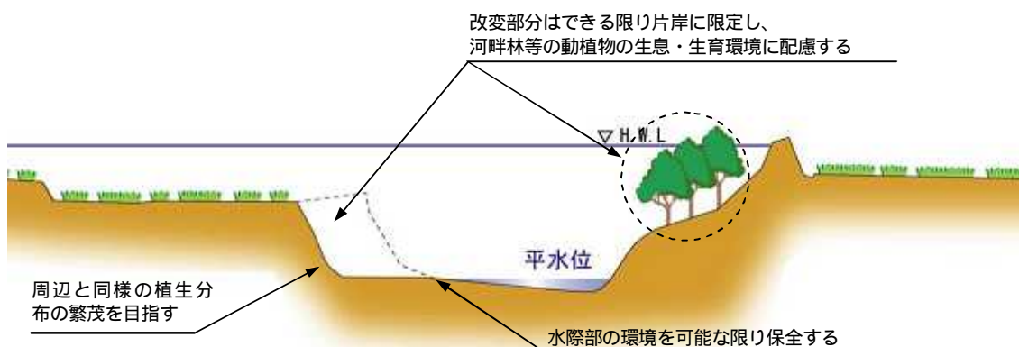
<多自然川づくり イメージ図>
