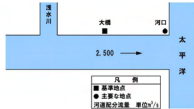
図 4.1 主要地点における河道配分流量
