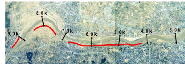
図 5.3 堤防の量的整備位置(平成 21 年 3 月時点)
