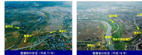
図 2.11 馬淵川の災害復旧事業概要
