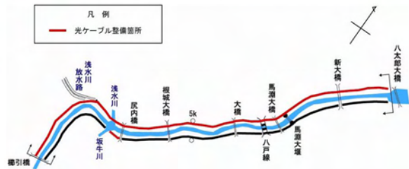
図 5.20 光ケーブルの敷設状況
