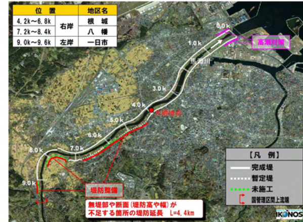
図 5.3 堤防の量的整備位置(平成 21 年 3 月時点)
