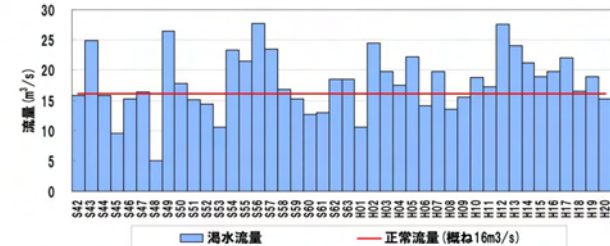
図 3.13 洪水流量の経年変化(剣吉地点)
