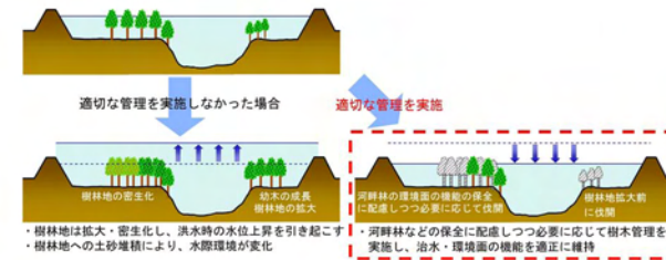
図 5.16 樹木管理のイメージ (断面図)
