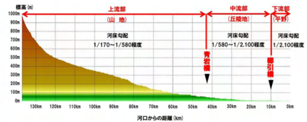
図 3.2 馬淵川河床勾配縦断面図
