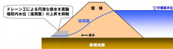
図 5.5 堤防の質的整備のイメージ
