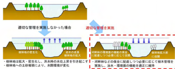
図 5.17 樹木管理のイメージ (断面図)
