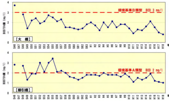
図 3.16 各環境基準点における水質経年変化(BOD75%値 ※ )
