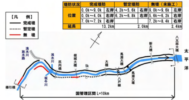
図 3.7 堤防整備状況
