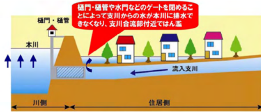
図 3.9 内水が発生する要因
