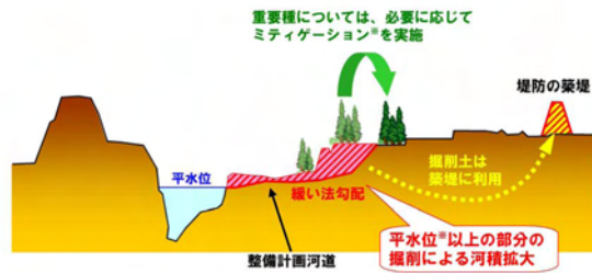
図 5.7 河道掘削のイメージ
