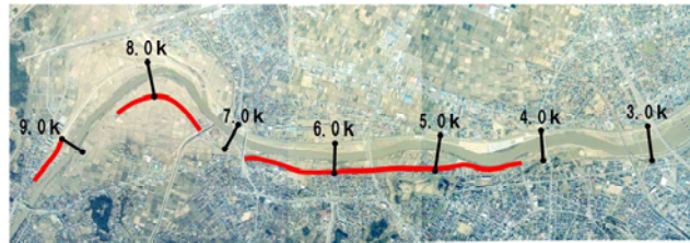
図 5.3 堤防の量的整備位置(平成 20 年 3 月時点)
