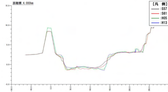
図 5.15 横断形状の経年変化 (河口より 4.0km 付近)
