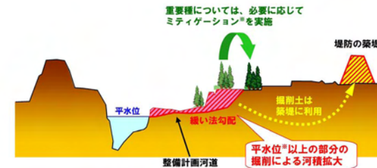
図 5.7 河道掘削のイメージ
