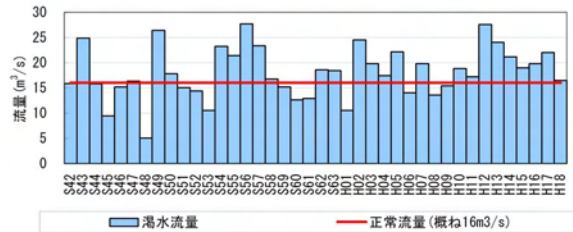
図 3.13 洪水流量の経年変化(剣吉地点)
