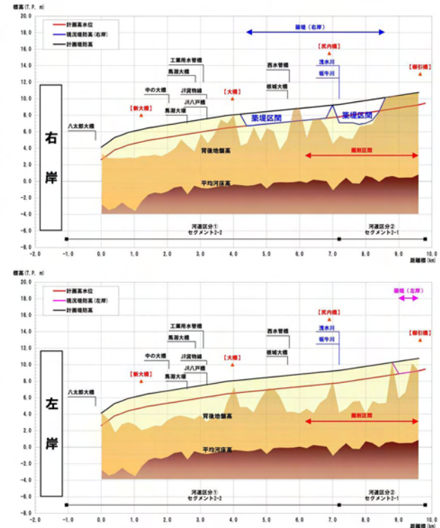
図 3.5 馬淵川の堤防整備縦断図 (平成 21 年 3 月 31 日時点)
