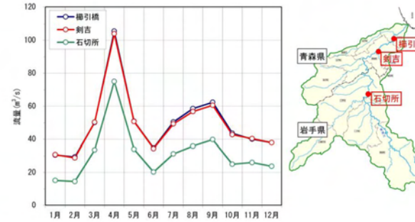
図 2.5 主要観測所地点の月別平均流量
