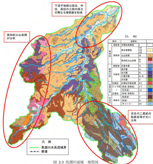
図 2.3 馬淵川流域 地質図
