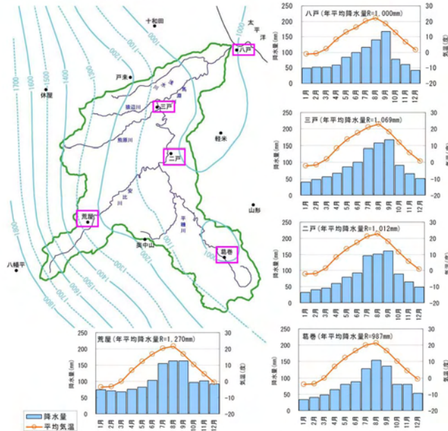
図 2.4 馬淵川流域 年降水量等雨量線図
