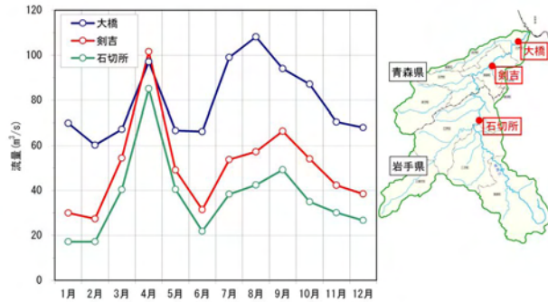
図 2.5 主要観測所地点の月別平均流量
