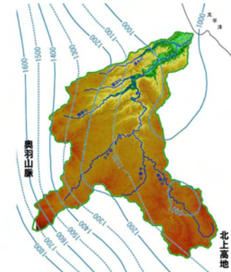
図 3.3 年降水量など雨量線図と馬淵川流域の地形
