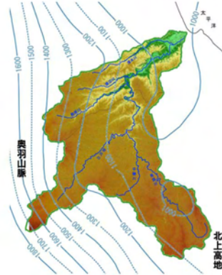
図 3.3 年降水量など雨量線図と馬淵川流域の地形
