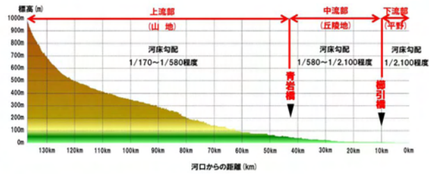
図 3.2 馬淵川河床勾配縦断面図
