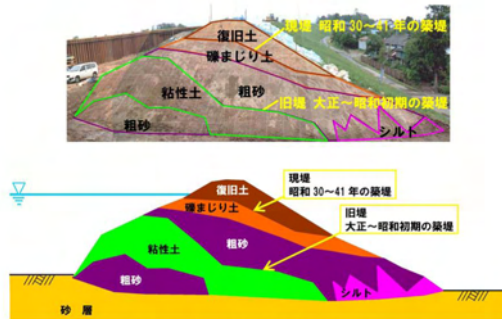
図 3.8 堤防及び基礎の土質イメージ
