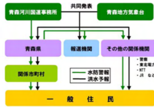
図 5.21 洪水予報・水防警報伝達経路
