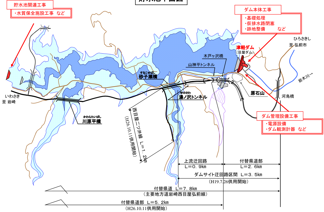
貯水池平面図
