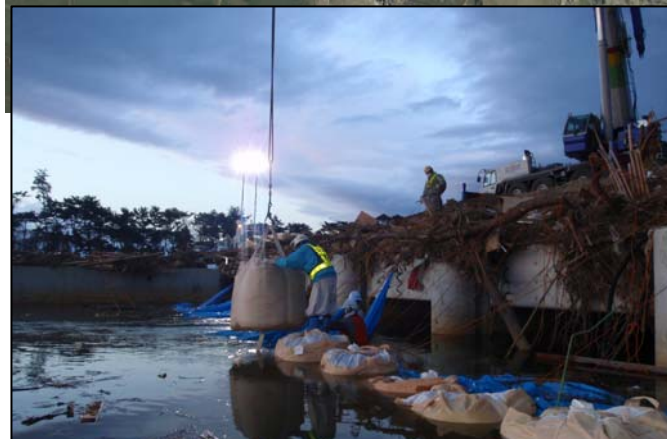
大型土のうによる締切作業(8日19時撮影)
