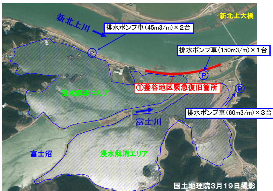
浸水解消のため、北上川右岸5k付近に排水ポンプ車を設置し排水作業を実施。(石巻市針岡地先)
