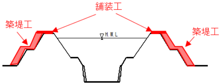
【断面図】
