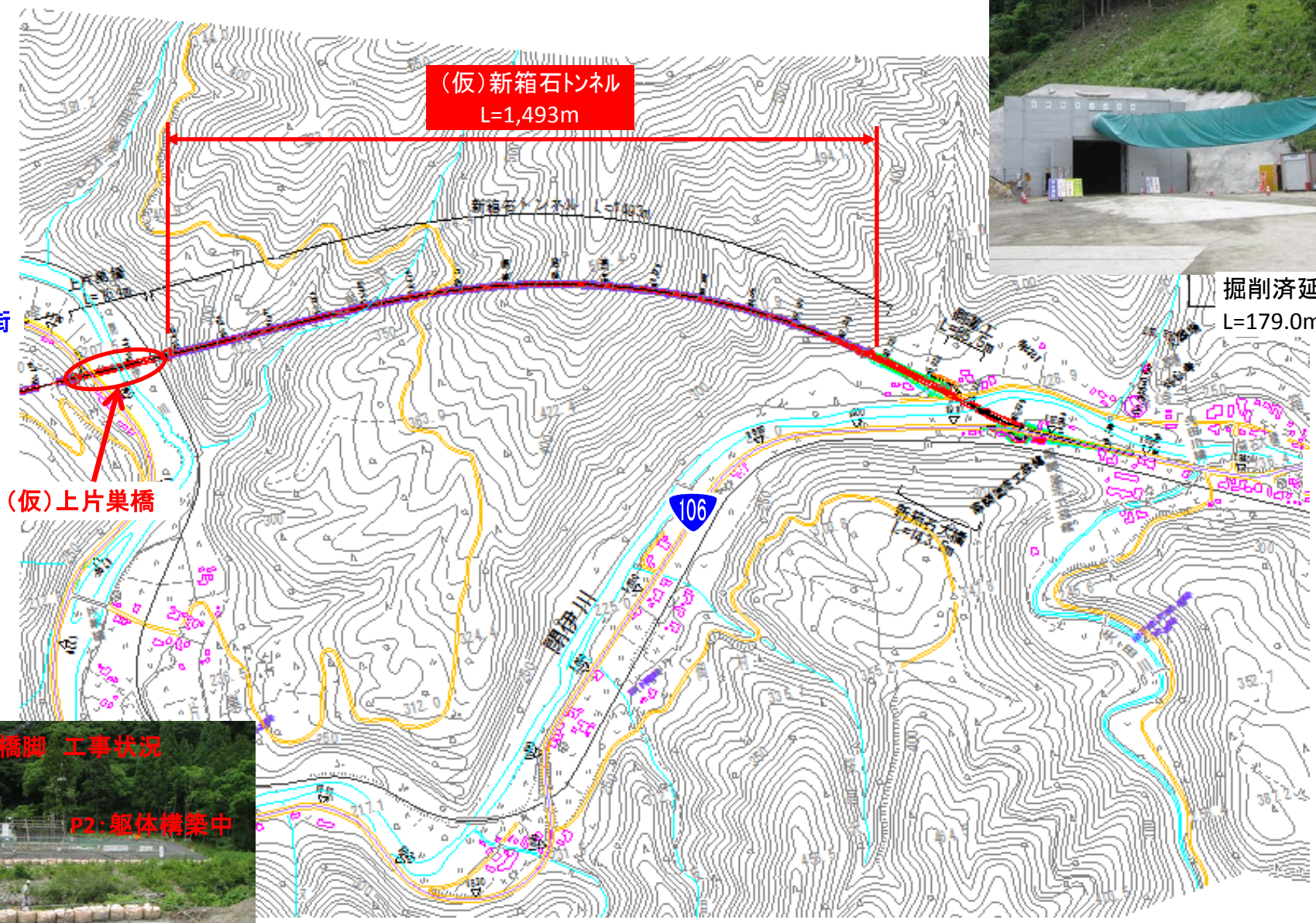
(仮)新箱石トンネル工事状況
