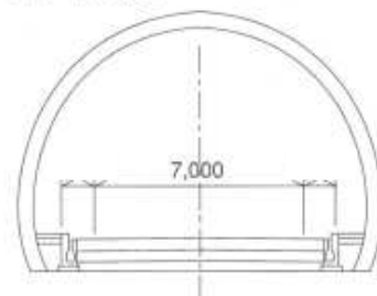
[トンネル部]
