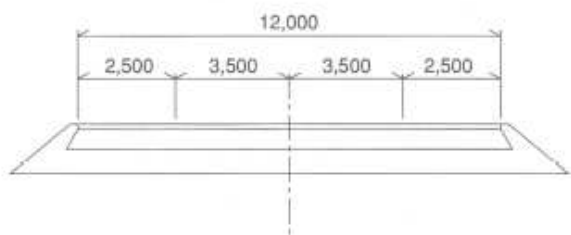
◆標準横断面 [土工部]
