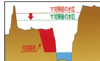
【河道掘削断面図】
