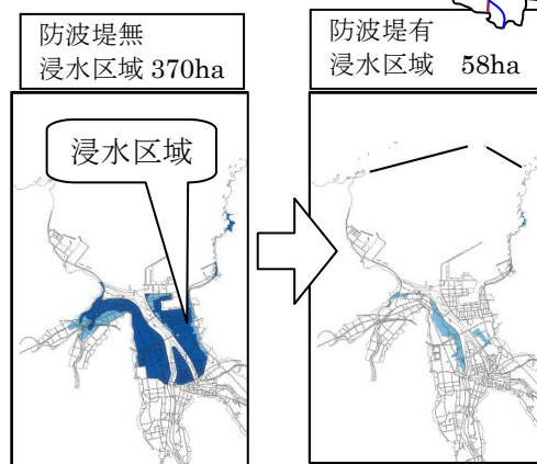
明治29年三陸津波によるシミュレーション（M8.5）
